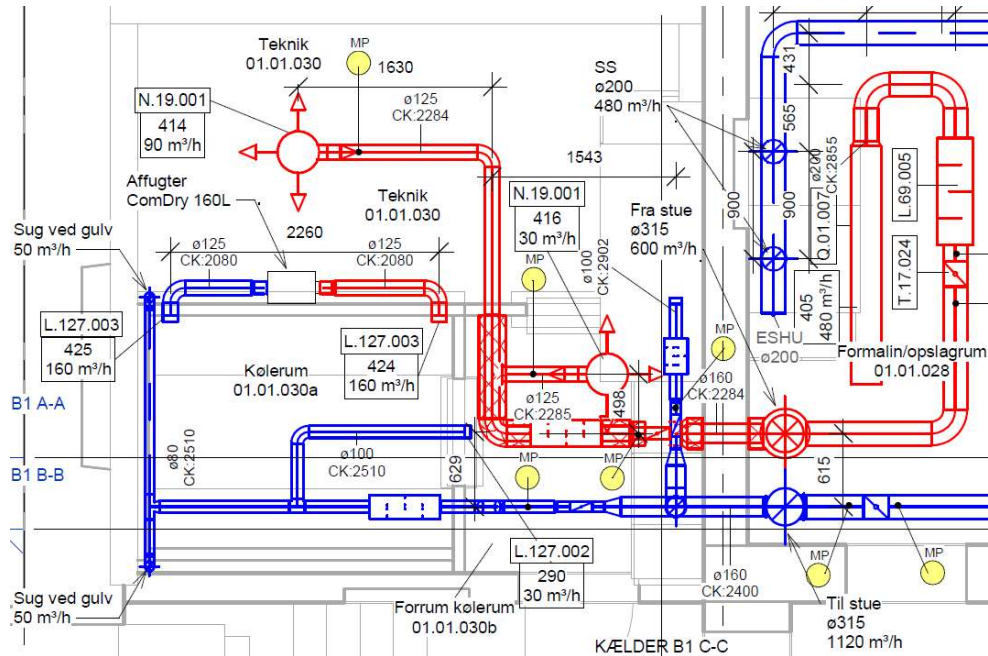
Illustration nr. 1 herover viser et eksempel fra arbejdstegninger, hvor luftmængder og målepunkter er angivet.
